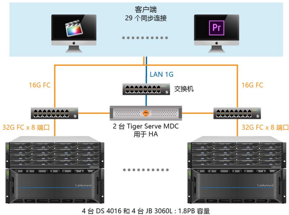
视频编辑应用的网络拓扑
